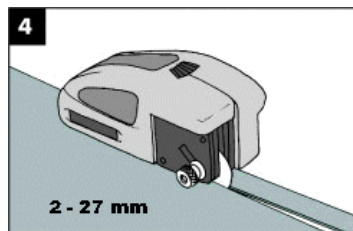
4 2 - 27 mm Schneiden von Intarsienstreifen
