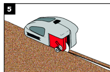
5 Nach dem Einsetzen der roten Distanzstücke ist das Unterschneiden einer Materialkante mit einer Neigung von 4 möglich. Nicht geeignet für das Schneiden von Wand zu Wand oder einem Doppelschnitt.
